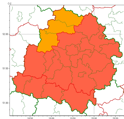
Burze z gradem 2023-08-26 20:56
