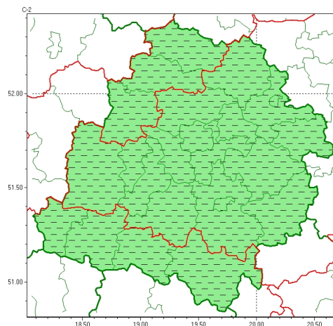
Silny deszcz z burzami 2023-08-26 20:56
